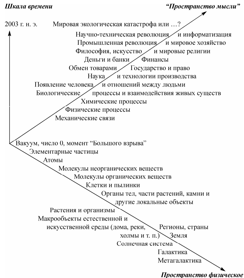
Рис. 1. Иллюстрация развития (развертывания) во времени объектов, субъектов и взаимосвязей физического и информационного пространств нашей Вселенной исходя из гипотезы “Большого взрыва”.
